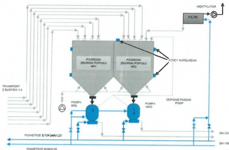
Rys 1. Schemat instalacji zbiornika pośredniego popiołu (wg Tymczasowej instrukcji eksploatacji elektrofiltrów 2022r.)
