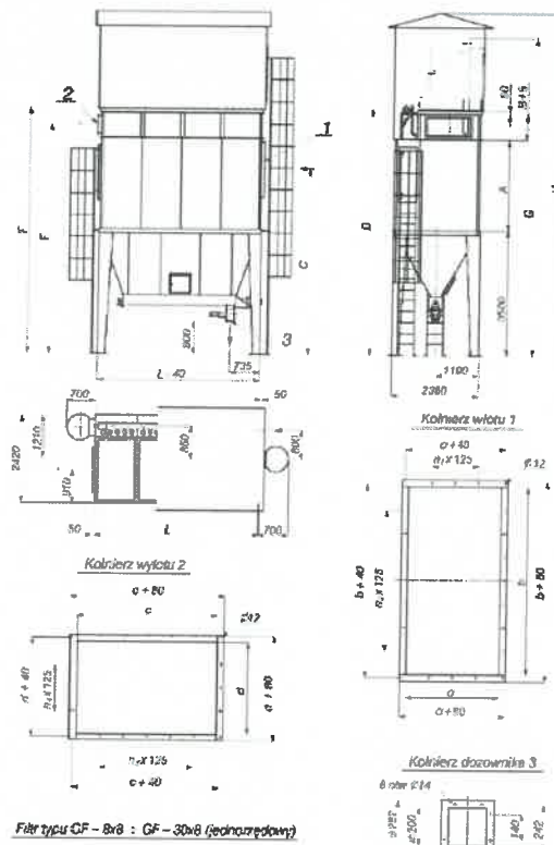
Rys 2. Poglądowy schemat filtra pulsacyjnego workowego typu GF (wymiary nie dotyczą filtra pulsacyjnego zainstalowanego na zbiorniku pośrednim na terenie zakładu ENEA Połaniec)
